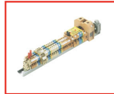
SAK 系列接线端子 SAK SERIES SCREW TERMINALS
